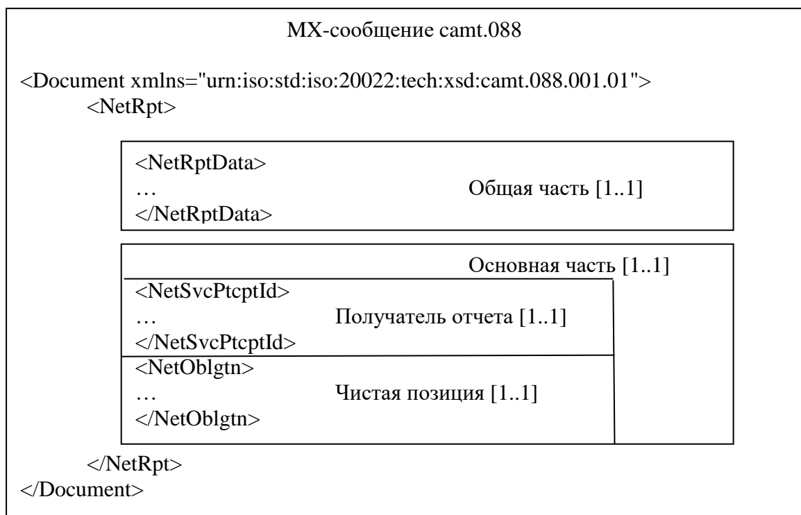
Рисунок 1 – Структура МХ-сообщения camt.088
